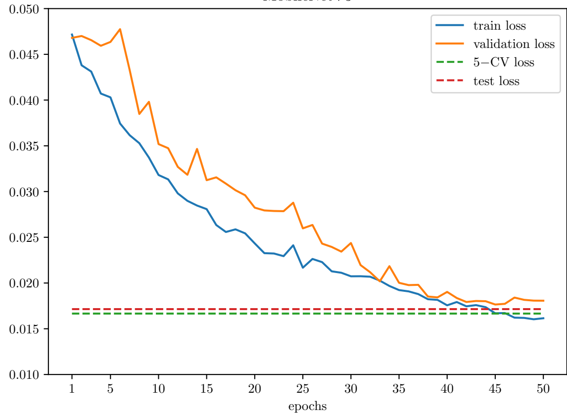
MobileNetV3
