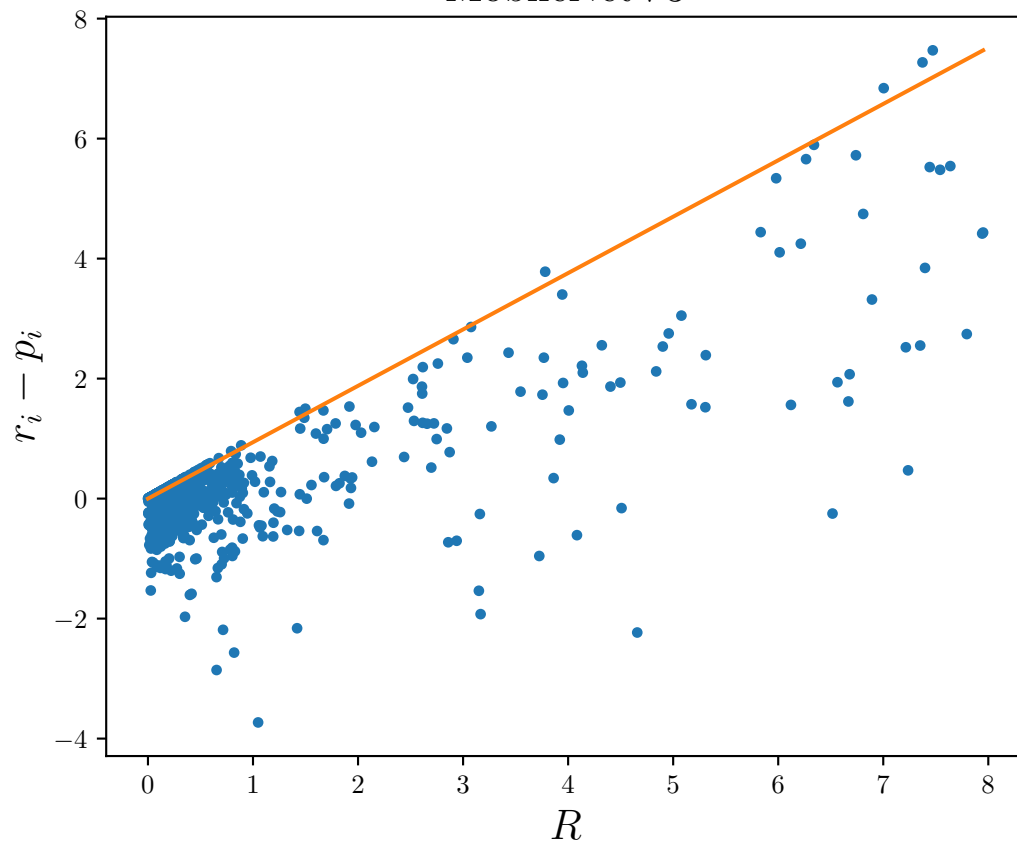
MobileNetV3
