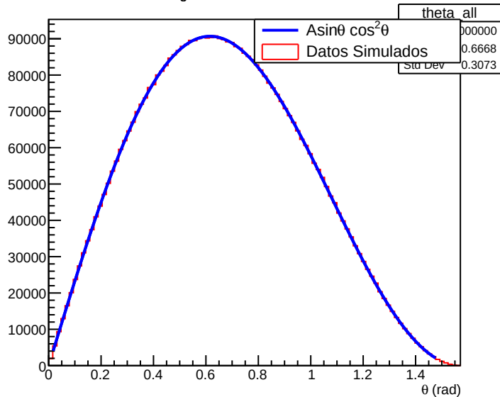
Distribución angular \theta de todos los muones simulados
