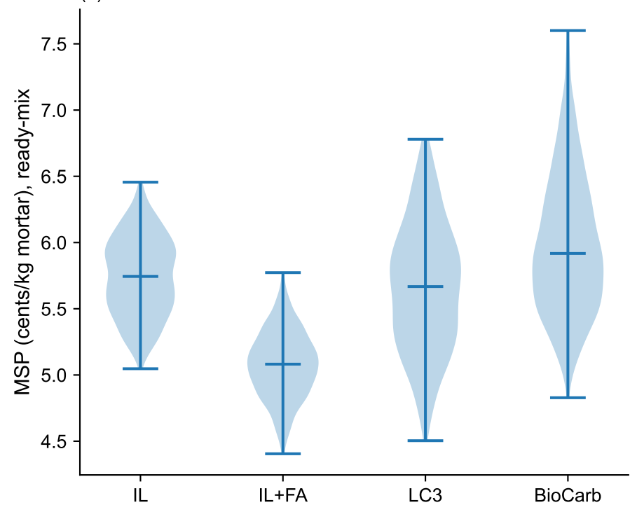
(d) Monte Carlo MSP
