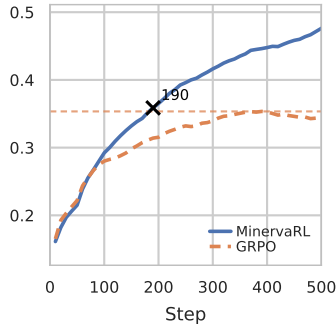
Llama-3.2-3B
