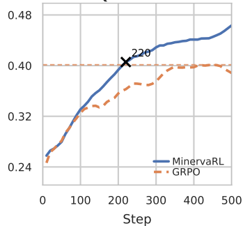
Qwen3-4B
