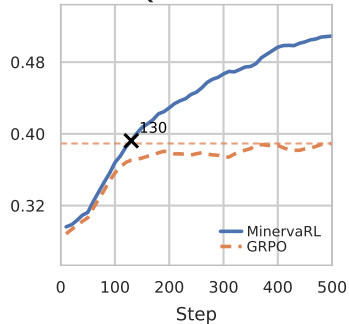
Qwen3-8B
