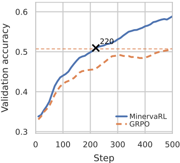
Llama-3.1-8B
