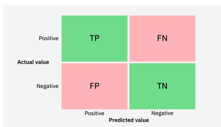
Figura 5: Matriz de confusão
