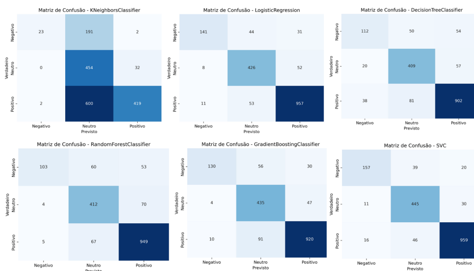
Figura 42: Matriz de confusão
