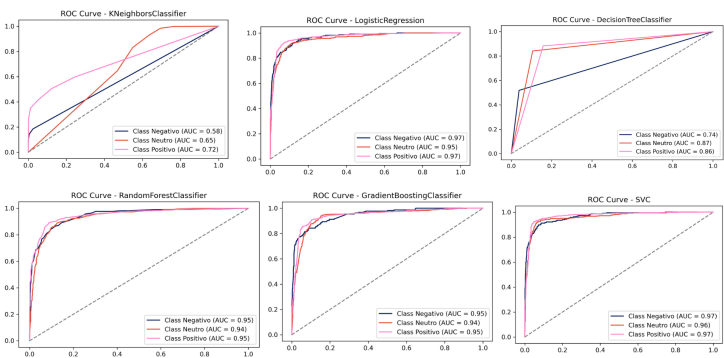
Figura 44: Curvas ROC de Desempenho dos Modelos
