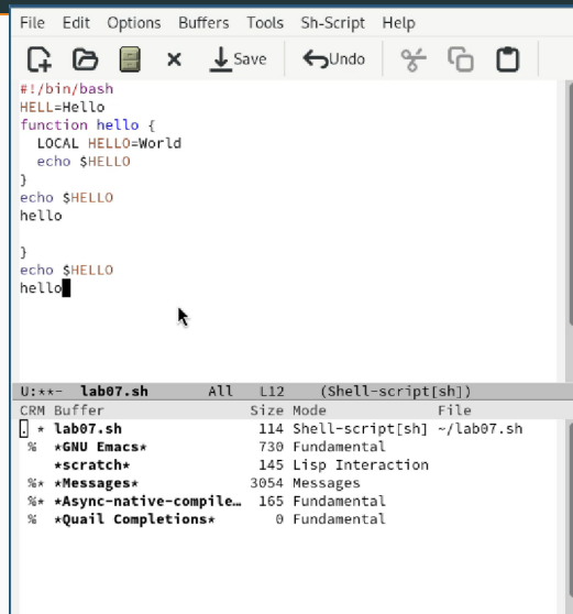
Рис. 14: Выводим список активных буферов на экран
