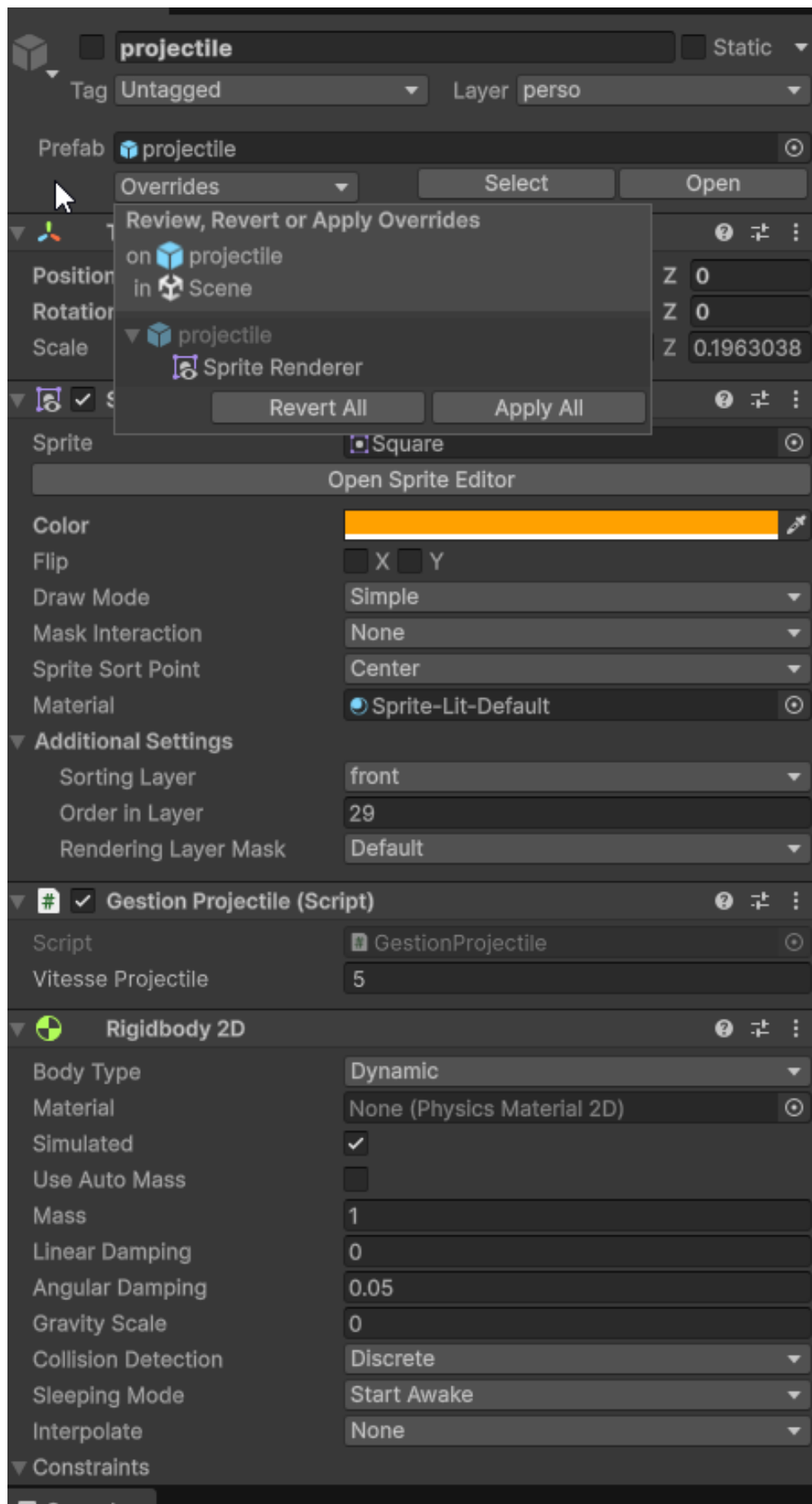
Figure 3 – Effacer les changements d'un prefab sur la scène
