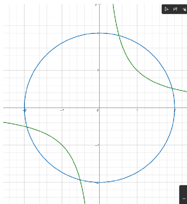
Рисунок 1 – Графики функций f_1(x, y) = 0 и f_2(x, y) = 0
