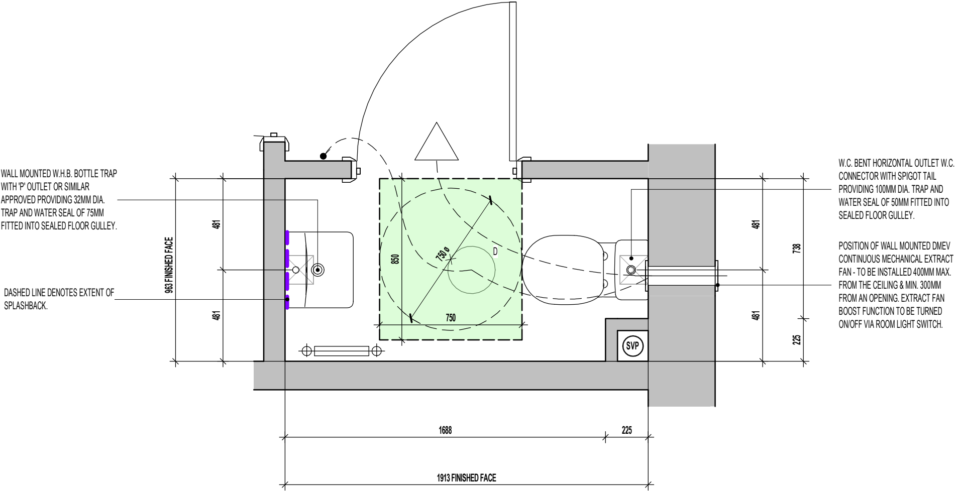
W/C LAYOUT SCALE : 1:20
