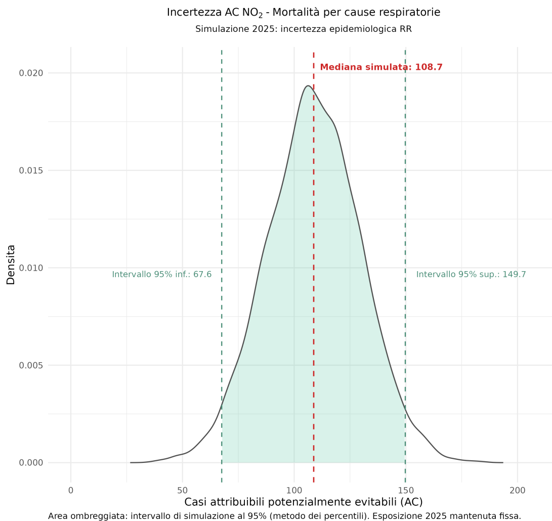
Figura 10: Distribuzione Monte Carlo dei casi attribuibili/anno per mortalità respiratoria nella popolazione 30+ della Regione Veneto nel 2025. Le linee verdi delimitano l'IC 95% propagato dall'incertezza epidemiologica del rischio relativo.
