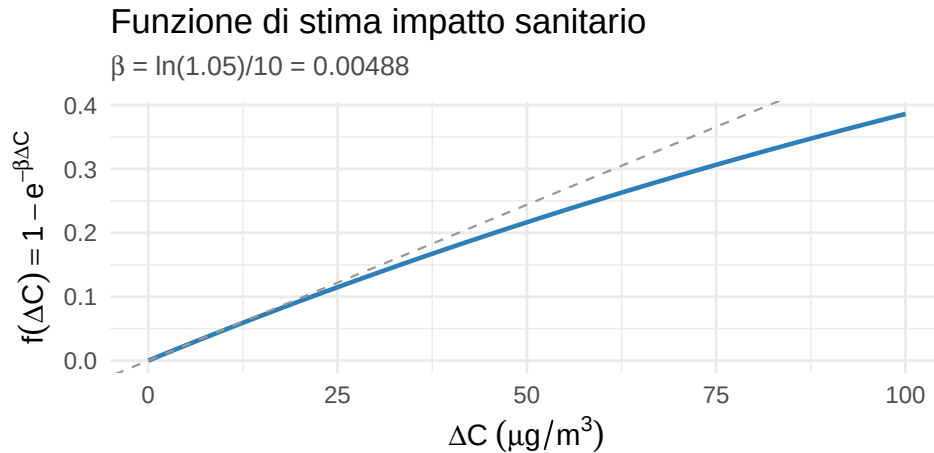
Figura 13: Funzione di stima dell'impatto sanitario in funzione di \Delta C
