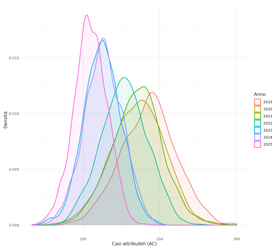
Figura 12: Distribuzioni dei casi attribuibili condizionate allo scenario annuale di esposizione NO_2 selezionato nella simulazione storica. Lo spostamento tra le curve riflette le differenze tra gli scenari di esposizione; la dispersione interna a ciascuna curva deriva dall'incertezza del rischio relativo.
