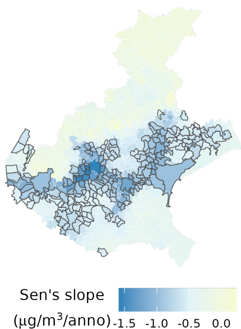
Figura 15: Trend annuale comunale di \text{NO}_2 (2019–2025). I colori rappresentano la pendenza di Sen; i bordi ispessiti identificano i risultati con p -value di Mann–Kendall aggiustato inferiore a 0,05.
