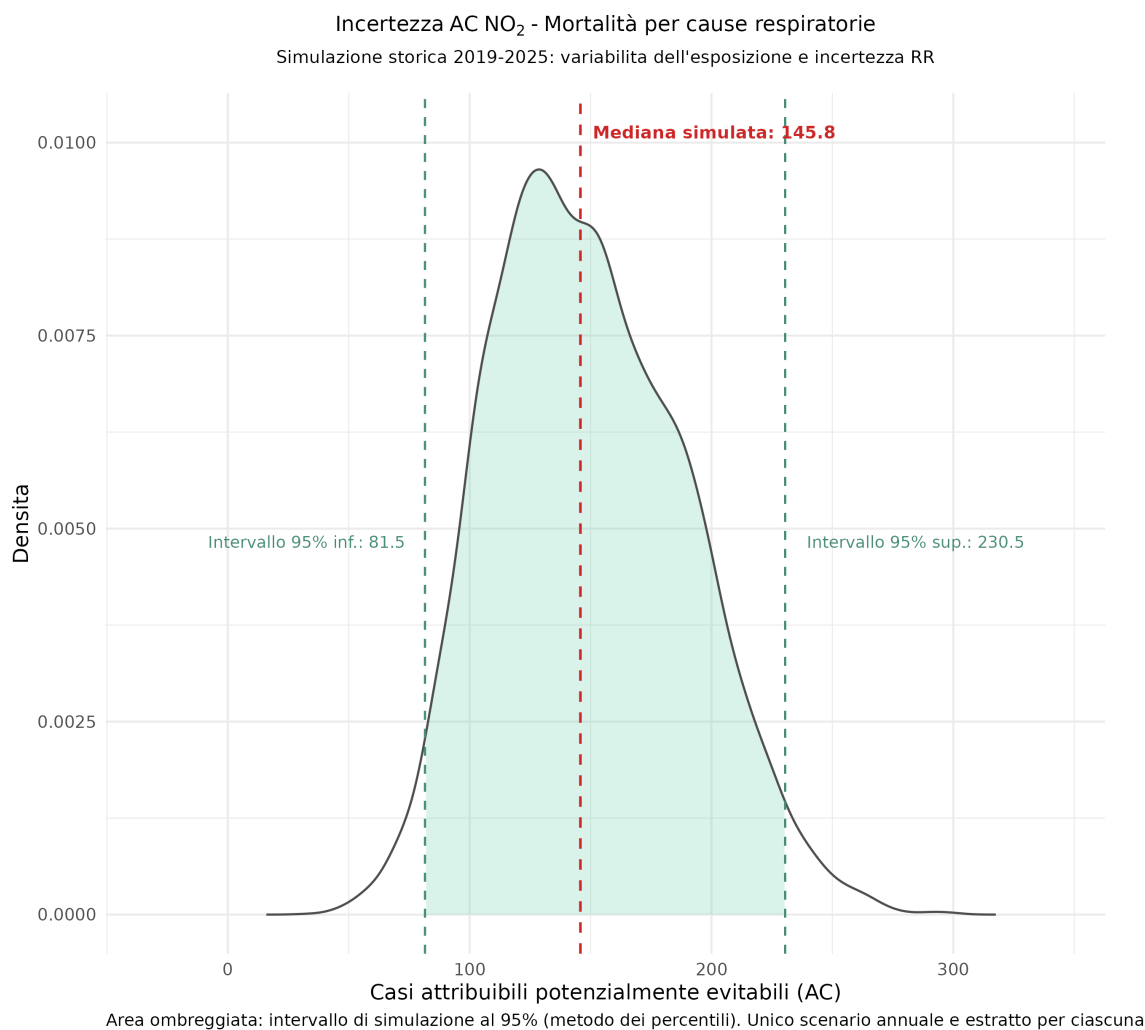
Figura 11: Distribuzione Monte Carlo dei casi attribuibili/anno ottenuta ricampionando gli scenari annuali di esposizione a NO_2 del periodo 2019–2025. Le linee verdi delimitano l’intervallo di simulazione al 95%.
