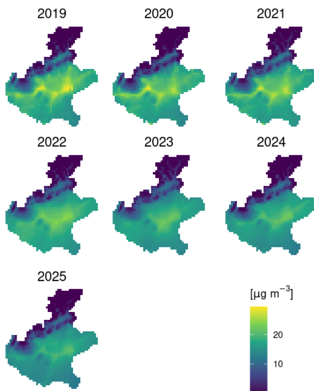
Figura 12: Serie storica concentrazioni NO_2 dal 2019 al 2025.
