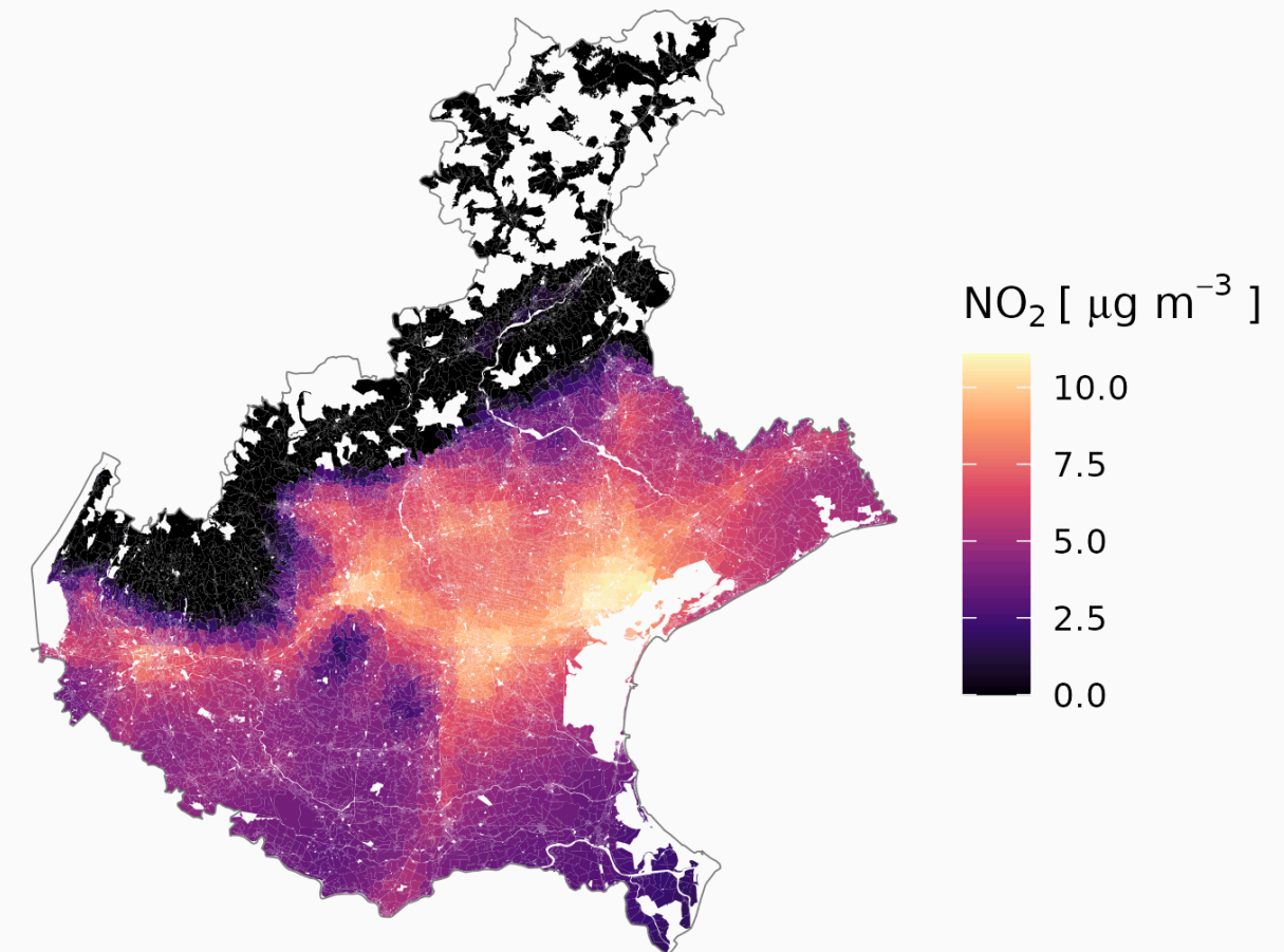
delta NO_2 : [2025] - [target OMS]
