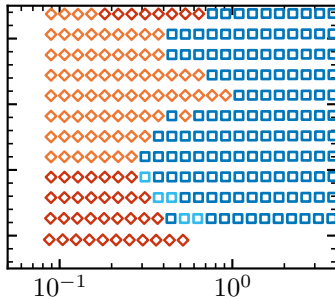
GRMHD
