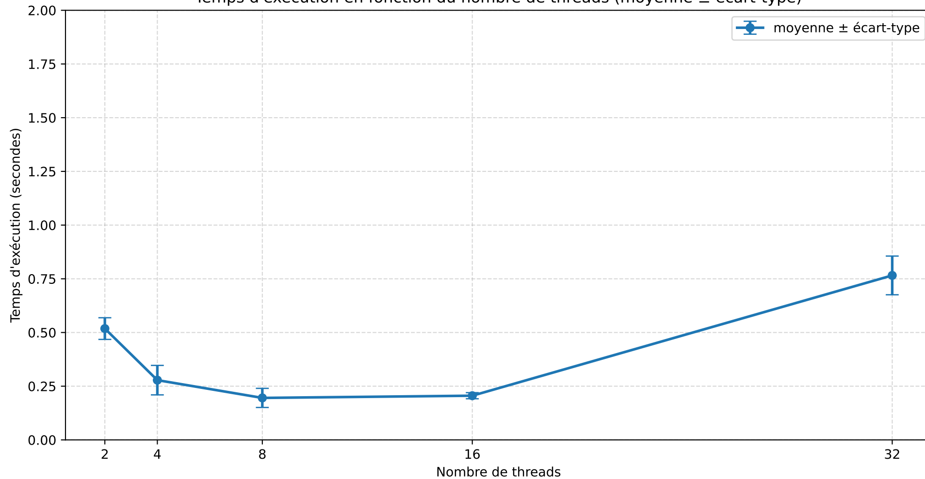
Temps d'exécution en fonction du nombre de threads (moyenne \pm écart-type)
