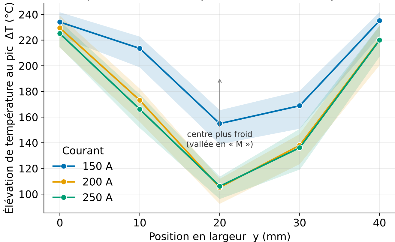
Profil de température en travers de la soudure (spot centré ; chants en y=0 et 40 mm, centre en y=20 )
