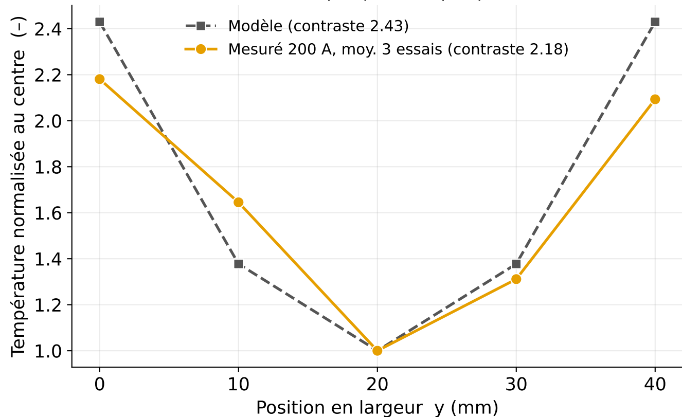
Le modèle reproduit la forme en « M » (contraste chant/centre un peu plus marqué que la mesure, 200 A)
