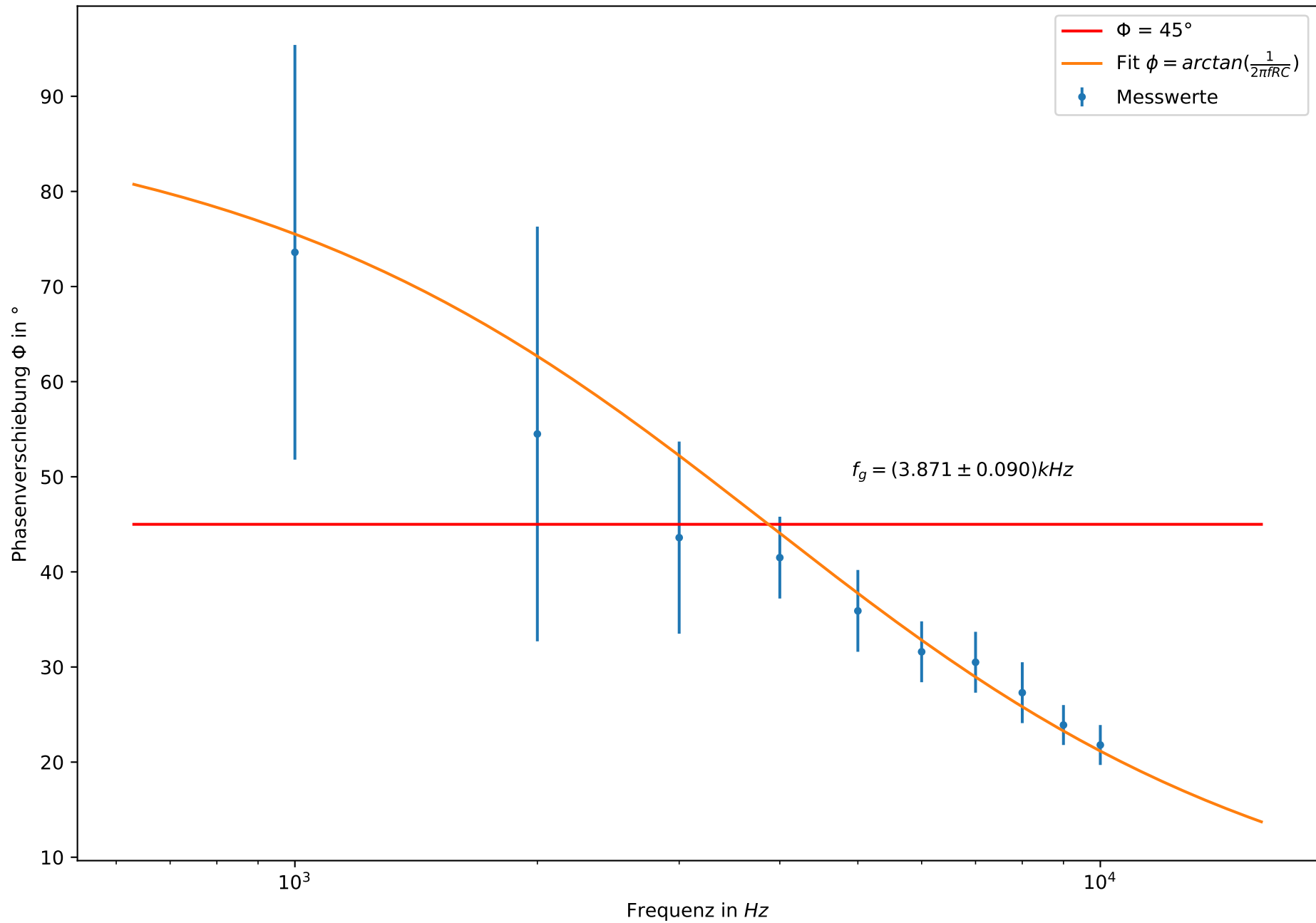
Diagramm 1 Phase gegen Frequenz für den Hochpassfilter
