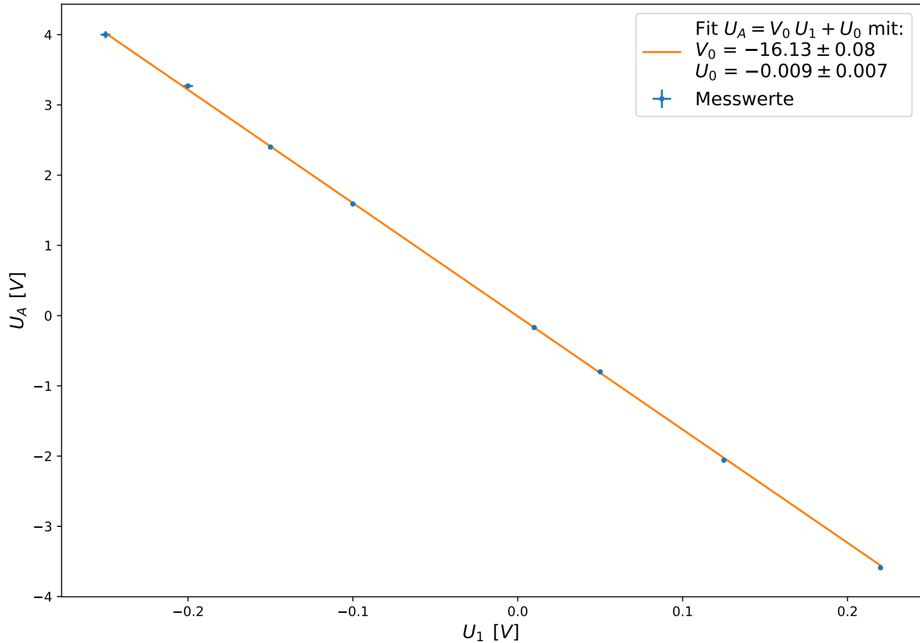
Ausgangsspannung U_A als Funktion von U_1 mit R_G = 48.7 \text{ k}\Omega
