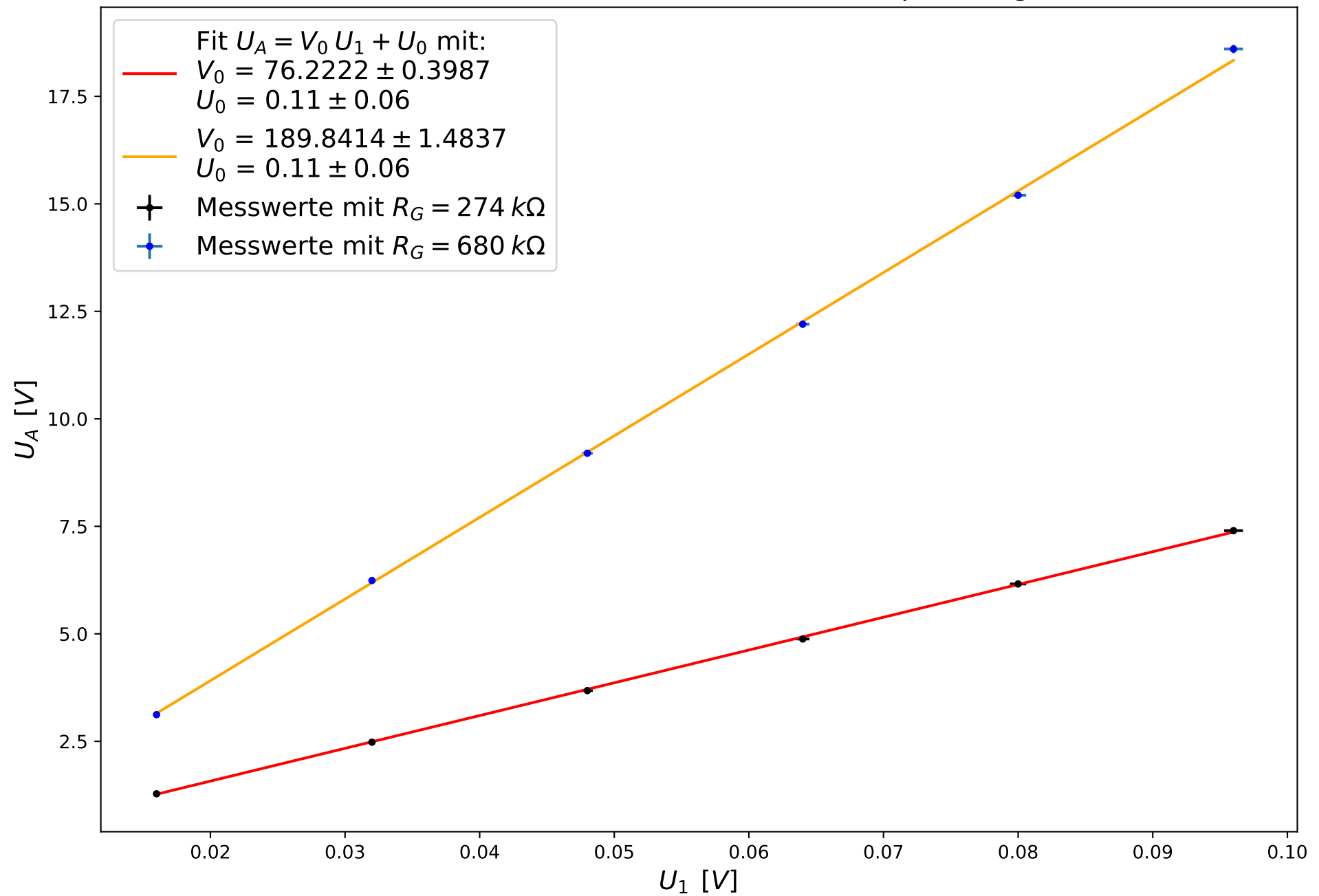
U_A als Funktion von U_1 bei Wechselspannung
