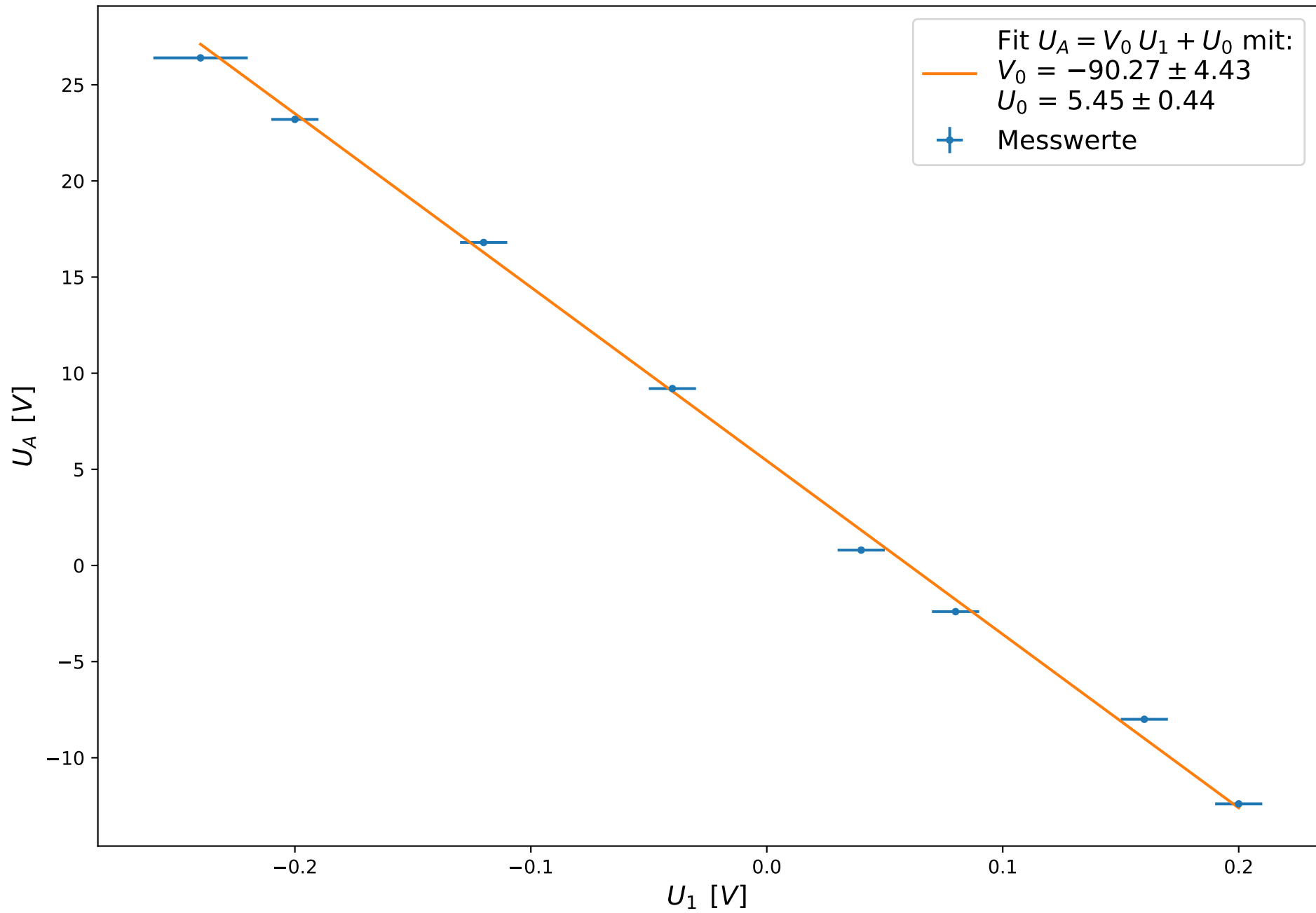
Ausgangsspannung U_A als Funktion von U_1 mit R_G = 274\text{ k}\Omega
