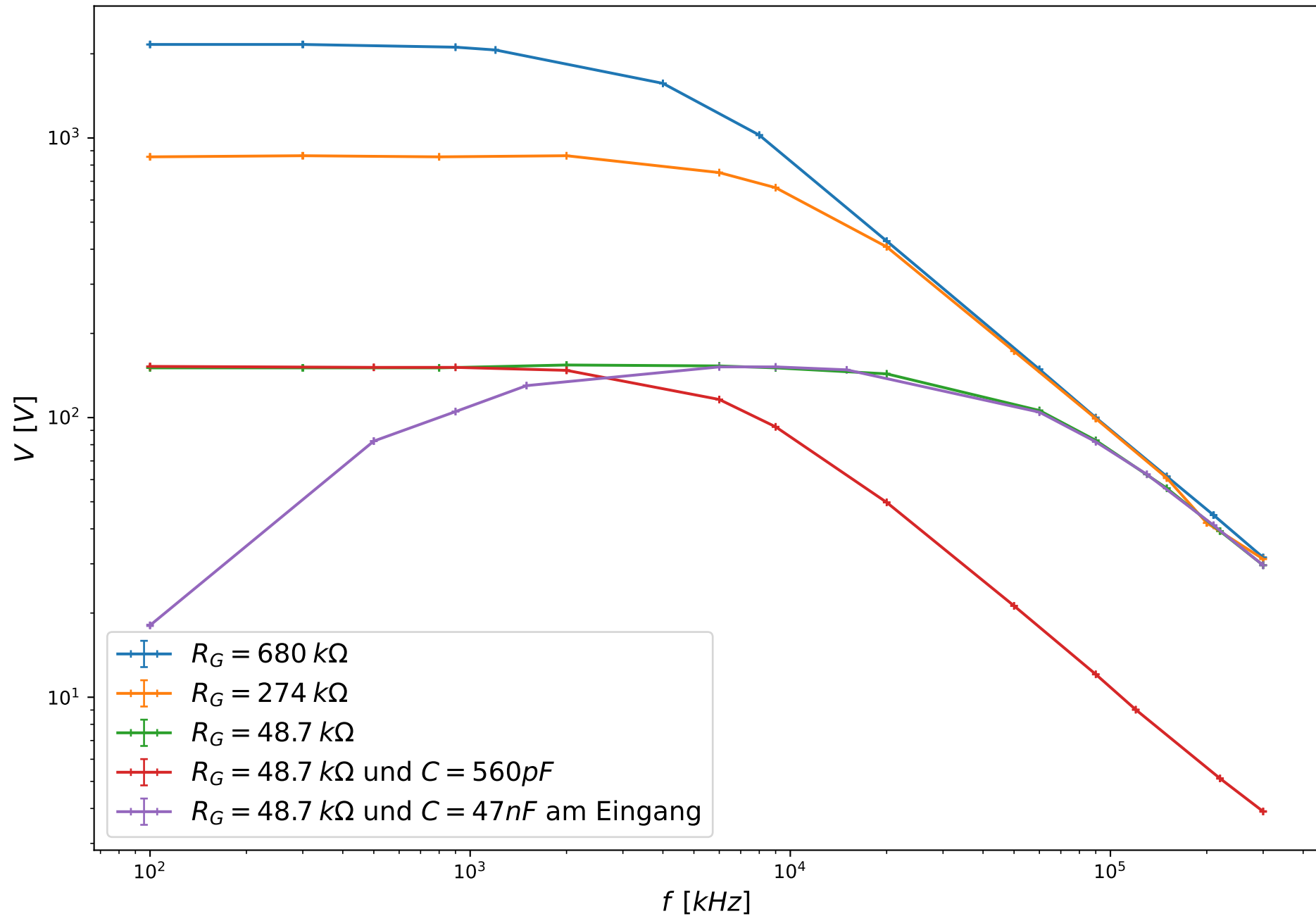
Frequenzgang des Verstärkers \mu A741 für verschiedene Gegenkopplungen
