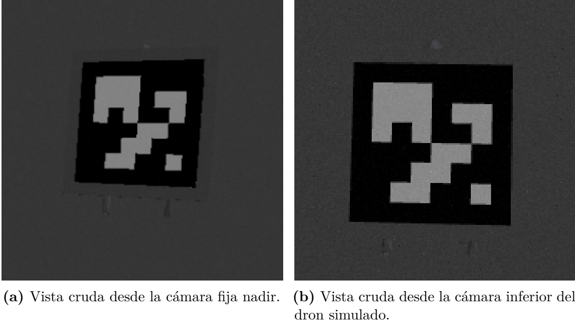
Figura 5.15: Comparación entre las dos fuentes de imagen empleadas en simulación para la estimación de pose del ArUco en tiempo real.
