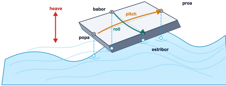
Figura 3.2: Esquema del efecto del oleaje sobre una embarcación: se identifican las cuatro zonas representativas de la cubierta (proa, popa, babor y estribor) y se sugiere cómo las diferencias de altura del agua bajo esos puntos se traducen en heave (traslación vertical neta), pitch (inclinación proa–popa) y roll (inclinación babor–estribor). Esta lectura motiva la aproximación discreta usada en el texto.
