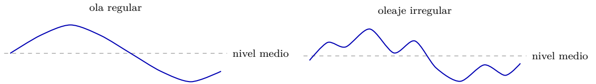
Figura 3.3: Perfiles conceptuales de la superficie libre. A la izquierda se presenta una ola regular con una escala temporal dominante. A la derecha se muestra una superficie más irregular representada como combinación de varias componentes.
