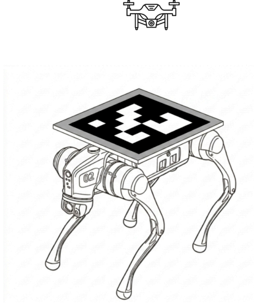
Figura 1.1: Esquema conceptual del montaje experimental base: Go2 instrumentado con tablero y marcador ArUco sobre el torso, junto con un dron ubicado por encima como referencia del escenario de observación aérea.
