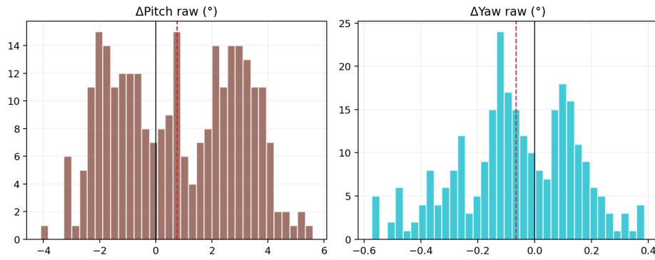
Figura 4.3: Distribución cruda del error angular en el caso base con cámara fija. Aquí se muestran \Delta pitch y \Delta yaw sin recentrado adicional, como apoyo para la lectura angular del caso base. La componente yaw se incluye solo como control diagnóstico, dado que el escenario no la excita deliberadamente. El histograma conserva el desfase temporal de la cadena de medición. Por eso debe leerse como error crudo y no como una distribución ya centrada en cero.
