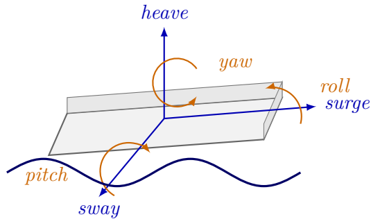
Figura 1.2: Convención de movimientos de plataforma marina usada en el trabajo. Se muestran los seis grados de libertad de una plataforma. Esta etapa prioriza roll , pitch y heave por su efecto directo sobre la observación visual del marcador.
