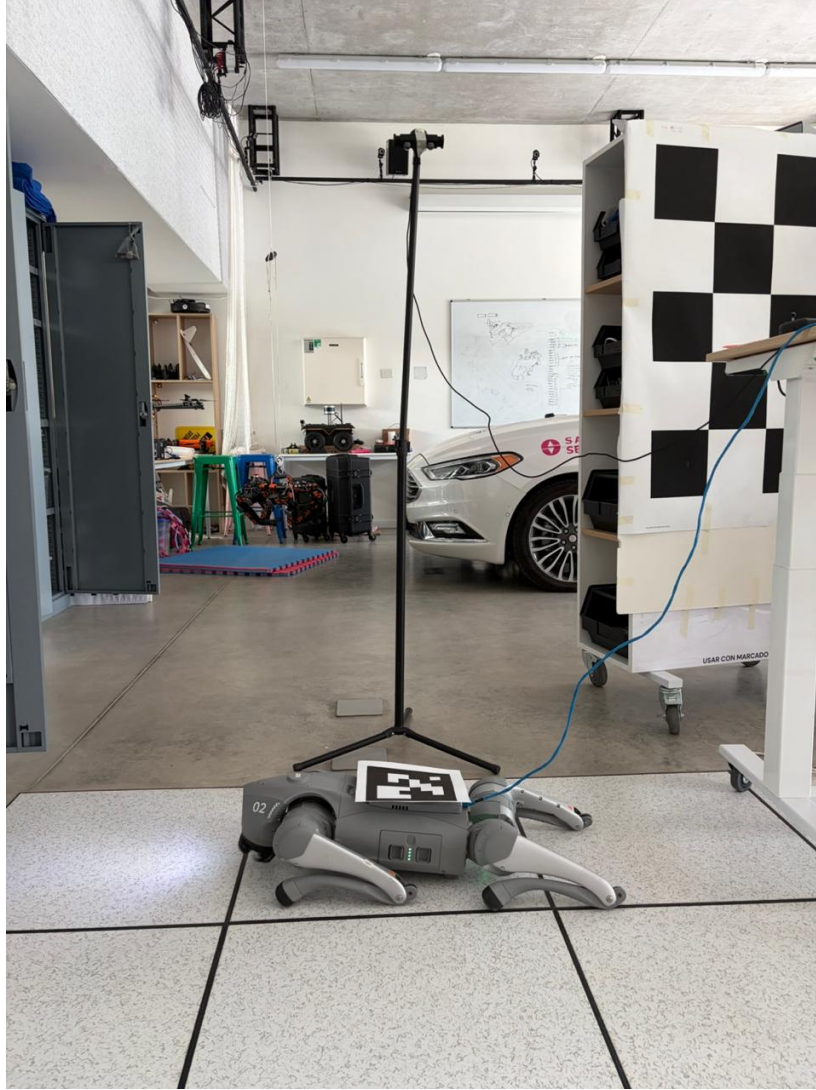
Figura 3.17: Geometría cámara–marcador del montaje de laboratorio: la cámara estéreo se mantiene aproximadamente fija sobre un trípode y observa el marcador ArUco adherido al torso del Go2. Esta disposición materializa la relación entre el plano del marcador y el marco óptico de la cámara utilizada por el método PnP para estimar pose en tiempo real.
