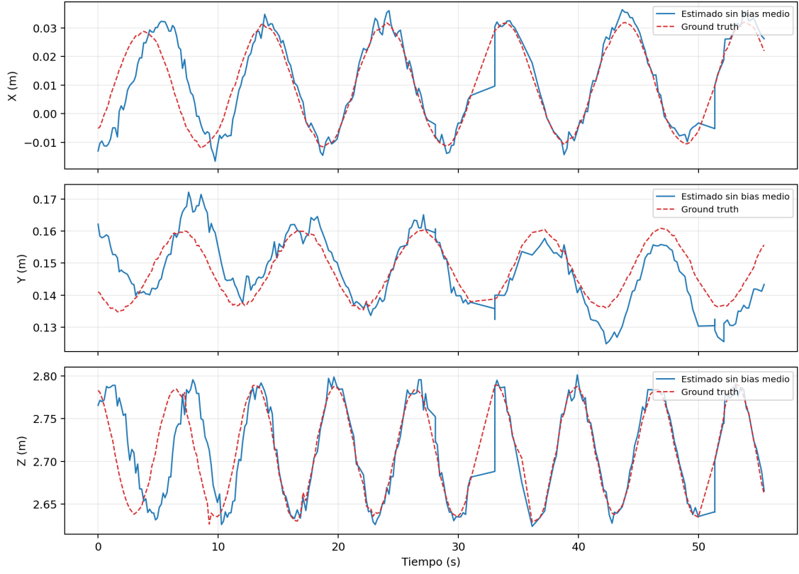
Figura 4.4: Comparación entre posición estimada y ground truth en la corrida principal del escenario con dron ( R2 ). La señal estimada se muestra sin sesgo medio por eje solo para visualización, de modo de facilitar la lectura de fase y forma temporal.
