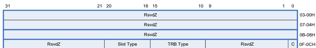
Figure 6-22: No Op Command TRB
