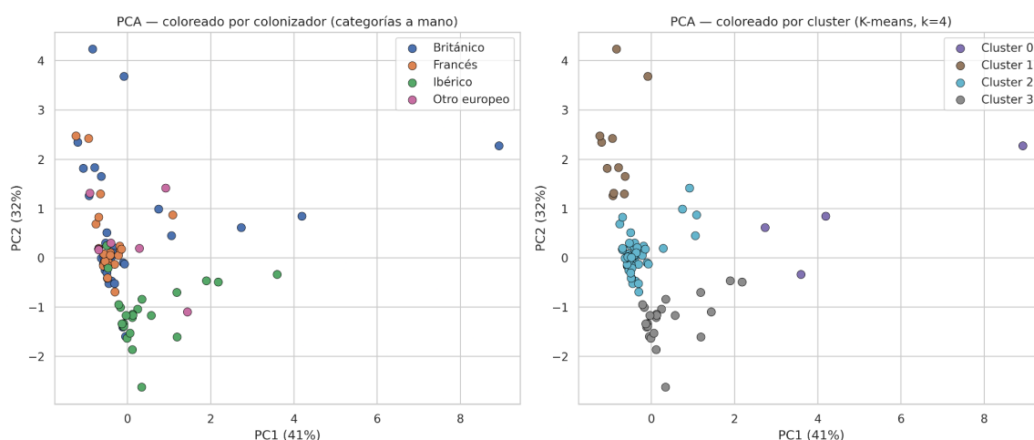
Fig 1. Gráfico de componentes principales. Colonizadores vs. Clúster K-Means.
