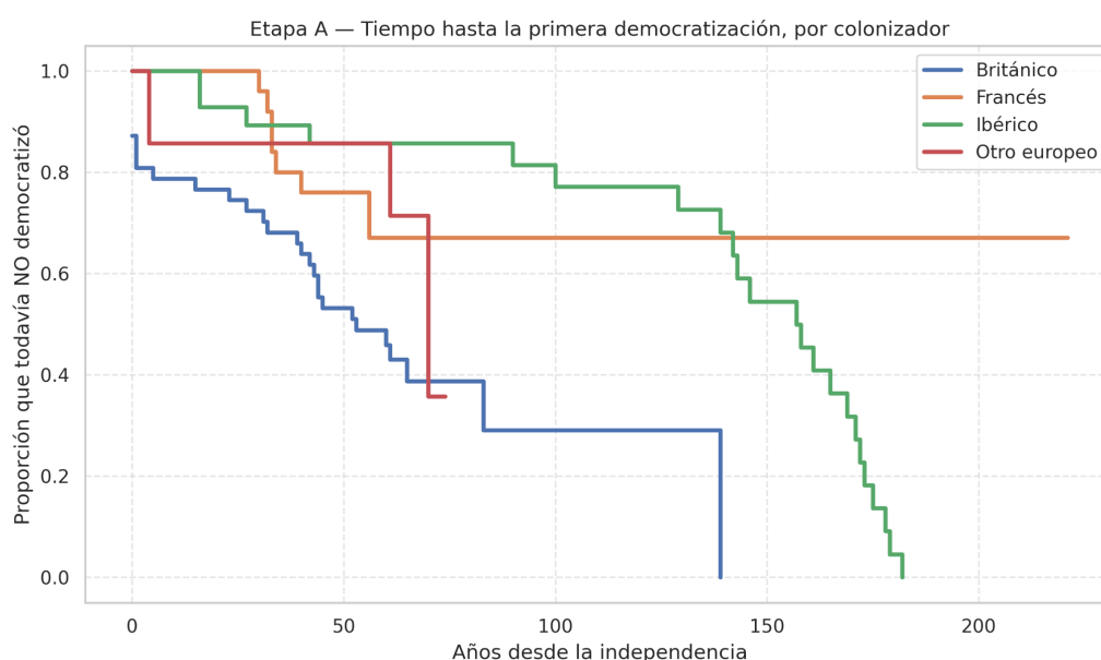
Fig 2. Curvas de Kaplan-Meier — tiempo hasta la primera democratización, por colonizador.
