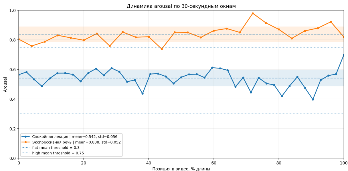
Рис. 3: Сравнение динамики arousal для спокойной лекции (V01) и экспрессивного выступления (V13). В экспрессивном примере средний arousal находится выше порога high ( \text{mean} = 0.838 > 0.75 ), поэтому срабатывает флаг эмоционального дисбаланса. В спокойной лекции среднее значение остаётся в нормальной зоне ( \text{mean} = 0.542 ), а вариативность невысока ( \text{std} = 0.056 ).
