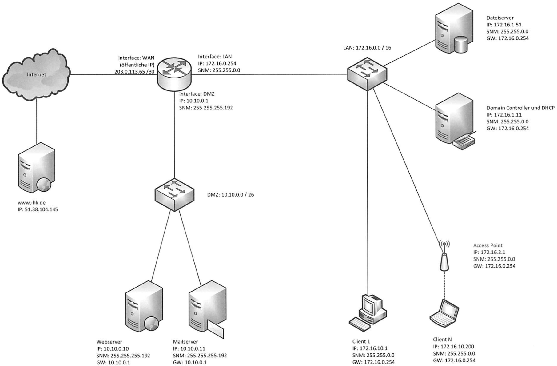
Anlage 1: Netzwerkplan der IHK-Multimedia-Agentur
