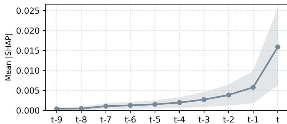
GgleReces
