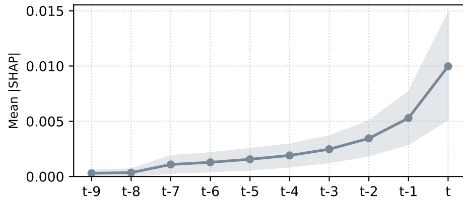
GeopolRisk
