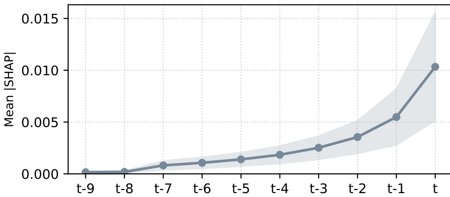
SP500
