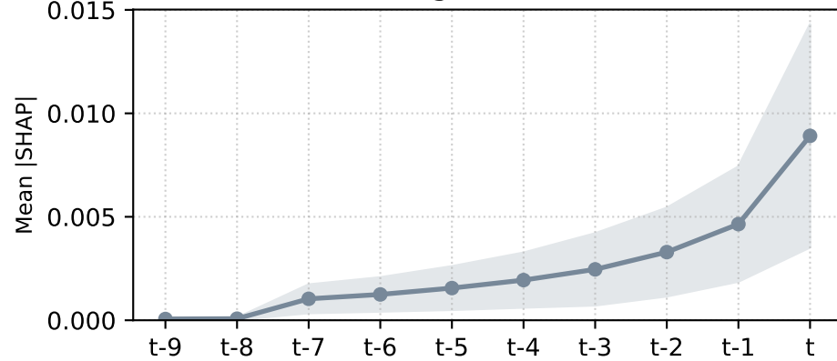
MPE
