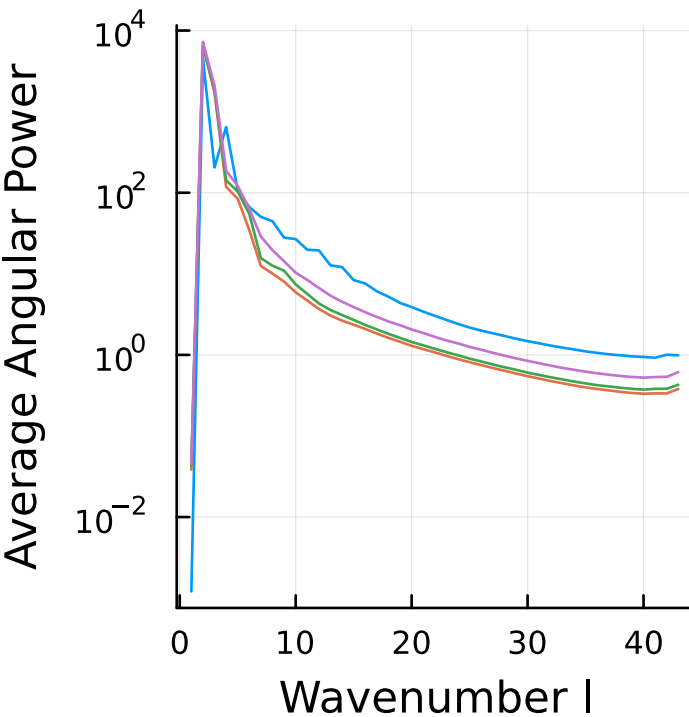
PS UNET 200 hPa
