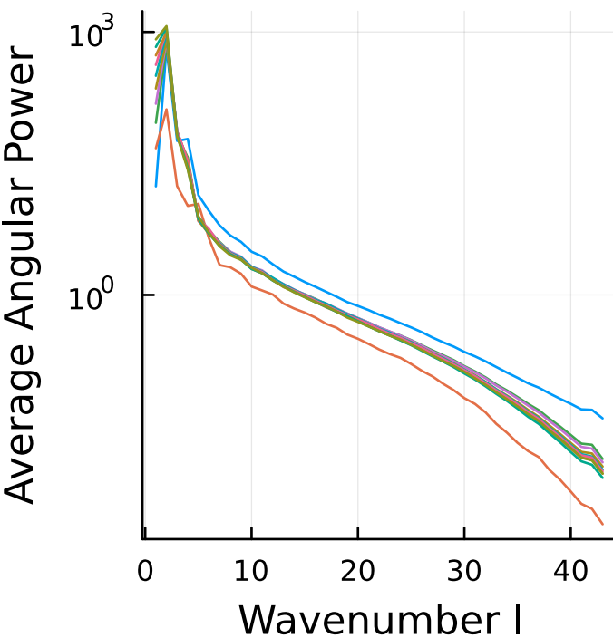
PS UNET 200 hPa
