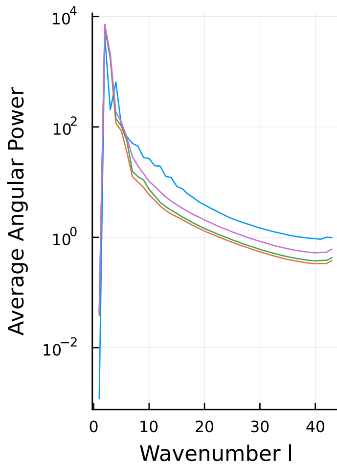
PS UNET 200 hPa
