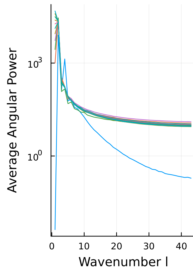
PS UNET 850 hPa
