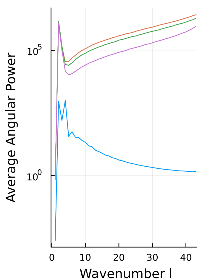
PS UNET 500 hPa
