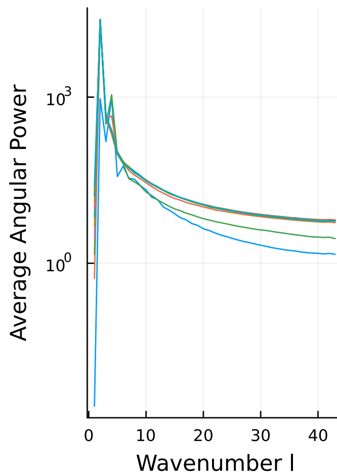
PS UNET 500 hPa
