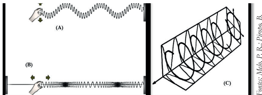
ILUSTRAÇÃO 3. (A) ONDAS TRANSVERSAIS. (B) ONDAS LONGITUDINAIS. (C) ONDAS CIRCULARES.
