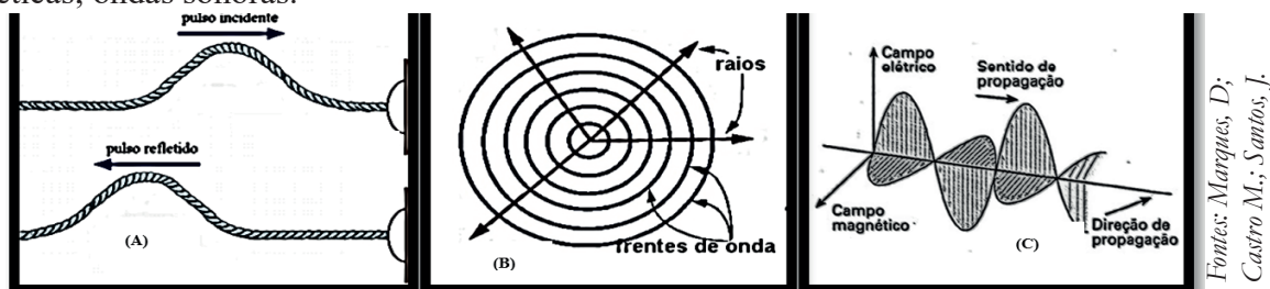
ILUSTRAÇÃO 4. (A) ONDAS UNIDIMENSIONAIS. (B) ONDAS BIDIMENSIONAIS. (C) ONDAS TRIDIMENSIONAIS.
