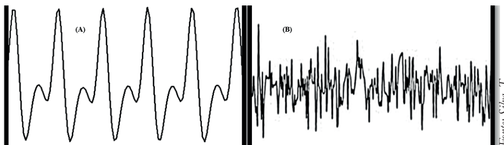
ILUSTRAÇÃO 5. (A) ONDAS PERIÓDICAS. (B) ONDAS APERIÓDICAS.
