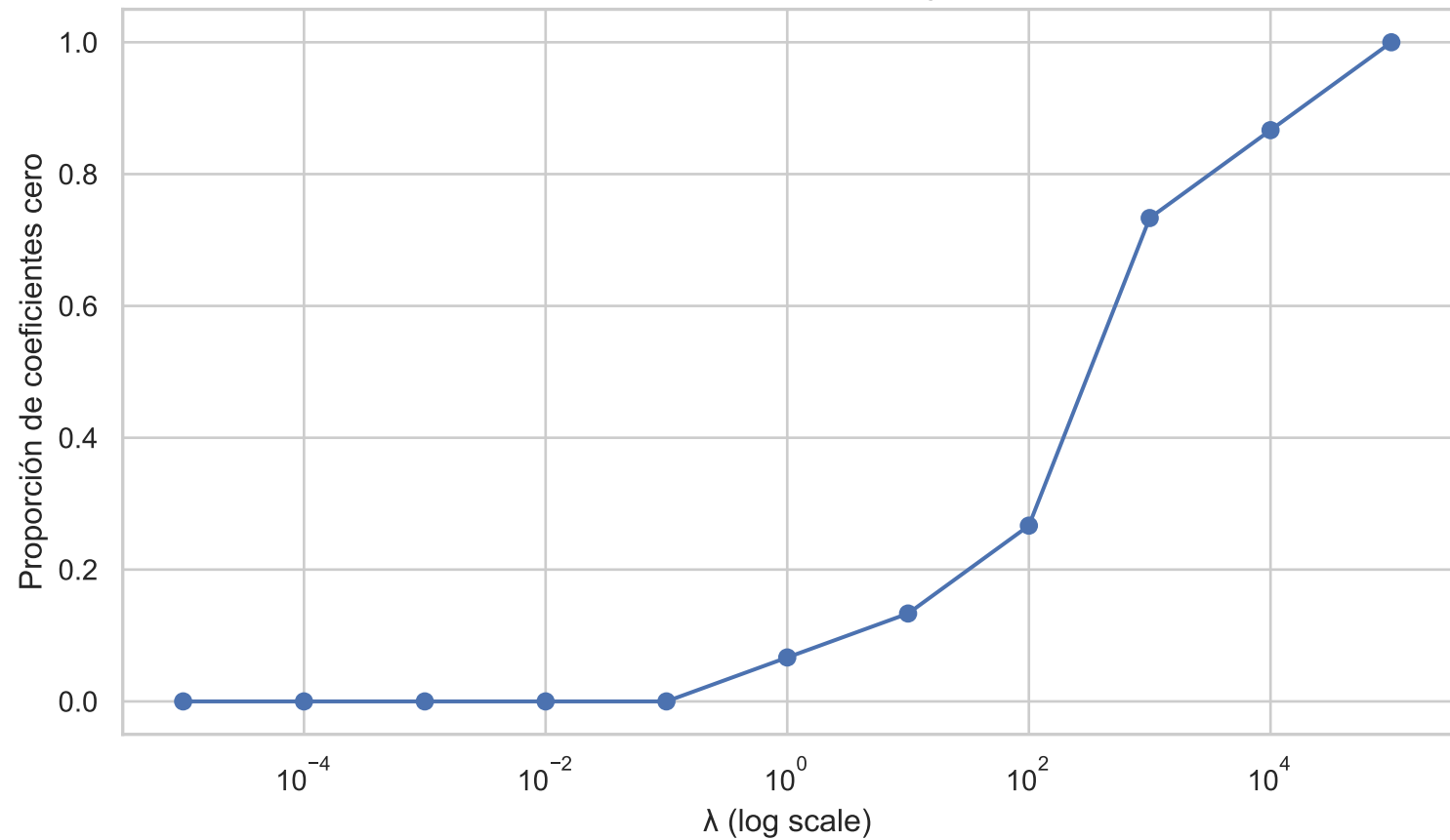
LASSO: Proporción de variables ignoradas vs \lambda
