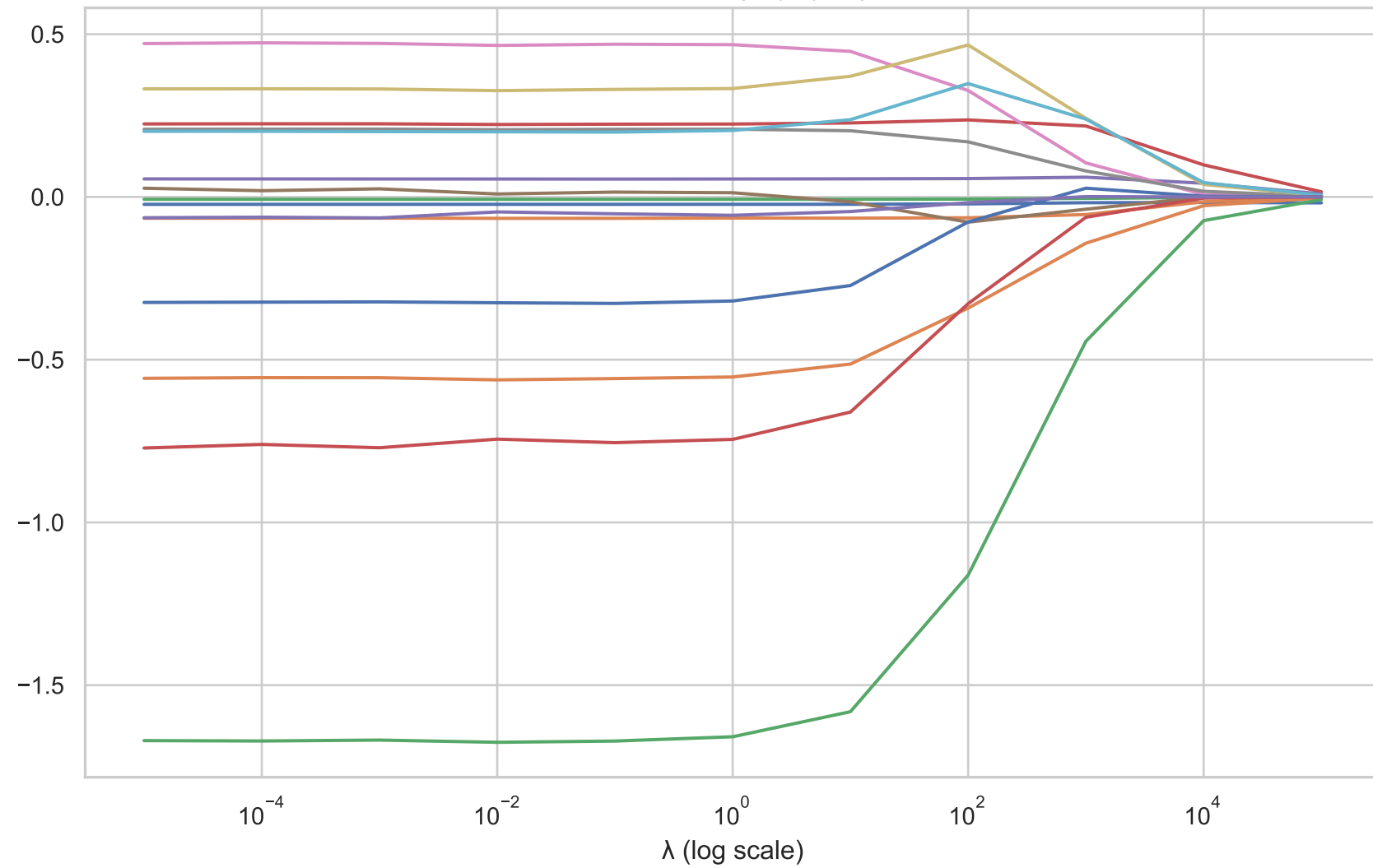
Coeficientes Ridge (L2) según \lambda
