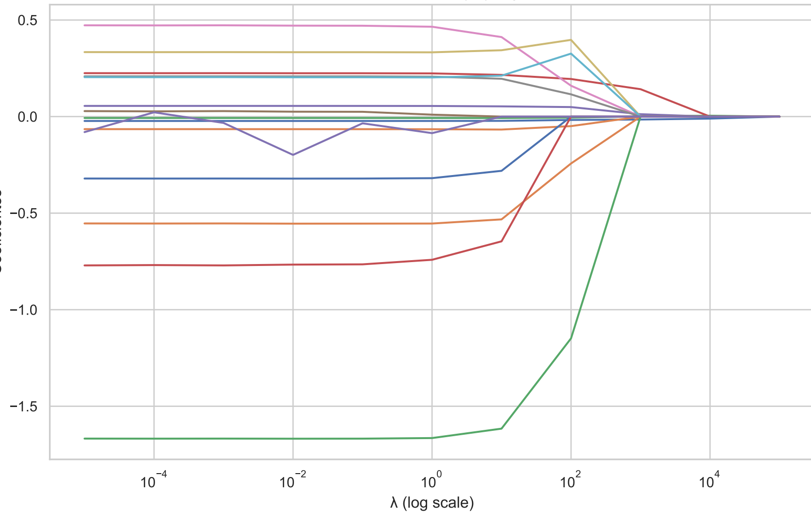
Coeficientes LASSO (L1) según \lambda
