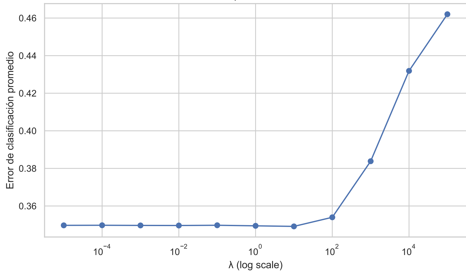
LASSO: Error promedio 5-fold CV vs \lambda
