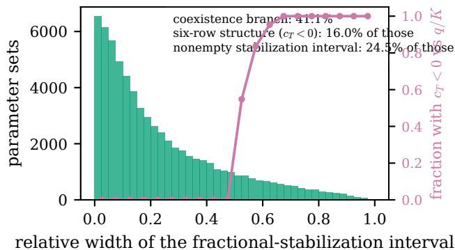
(d) ensemble of 10^6 random parameter sets
