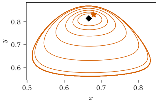
(d) surrogate phase portrait, \varepsilon = 0.05
