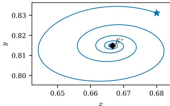
(d) surrogate phase portrait, \varepsilon = 0.05
