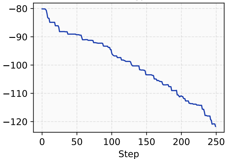
Dirac gap
