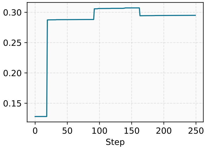
Dirac gap
