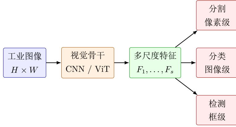
图 12.1: 视觉系统先由卷积或 Transformer 骨干提取表示，再按标签粒度输出分类、检测或分割结果。
