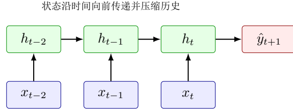
图 11.1: 递归序列模型把历史压缩为状态；状态维度和更新机制决定哪些信息能够持续保留。
