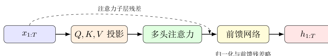
图 11.3: Transformer 编码块的主要信息流。
