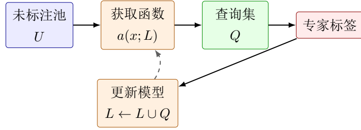
图 20.1: 池式主动学习在每轮用获取函数分配有限标注预算，再用新标签更新模型和下一轮查询。
