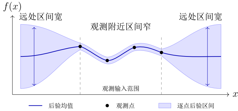
图 10.1: 高斯过程不确定性示意：观测附近的后验区间较窄，远离观测后逐渐变宽。
