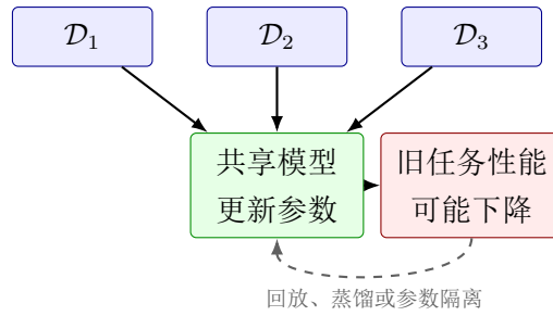
图 17.1: 持续学习沿数据流更新模型；新任务的可塑性与旧任务的稳定性形成直接张力。
