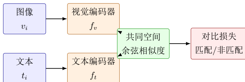
图 12.1: 双塔对比学习先把不同模态映射到共同空间，再用配对关系约束表示距离。
