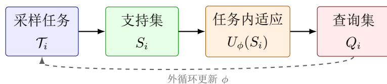
图 21.1: 元学习的双层结构：支持集用于适应，查询集评价适应后的模型并更新元参数。
