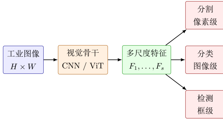
图 10.1: 视觉系统先由卷积或 Transformer 骨干提取表示，再按标签粒度输出分类、检测或分割结果。
