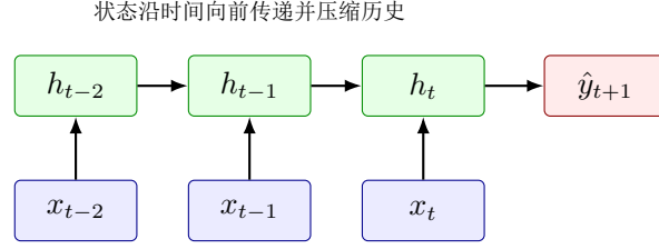
图 9.1: 递归序列模型把历史压缩为状态；状态维度和更新机制决定哪些信息能够持续保留。
