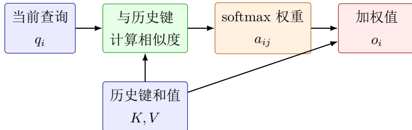
图 9.2: 注意力把“压缩全部历史”改为“按查询重新读取历史”, 代价是保存和计算位置间的相互作用。
