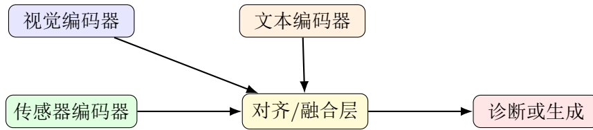
图 12.2: 工业多模态系统中，编码、对齐、融合和任务输出是不同层次。
