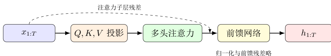
图 9.3: Transformer 编码块的主要信息流。
