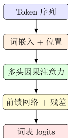
图 11.1: 自回归语言模型的基本计算链条。
