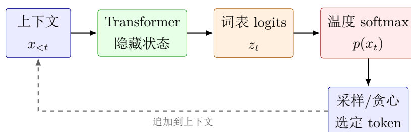
图 11.2: 自回归解码的单步迭代：模型先形成词表分布，再把选中的 token 反馈给下一步。
