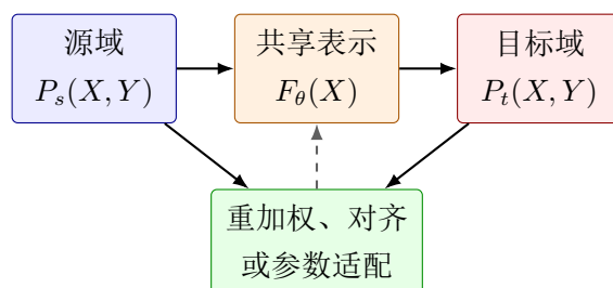
图 16.1: 迁移学习的核心是把源域知识送入目标域，同时检验哪些分布或任务假设仍然成立。
