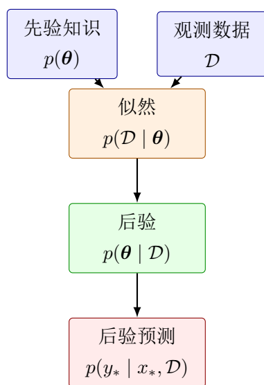
图 7.1: 贝叶斯更新把先验与观测结合为后验，再对参数不确定性积分得到预测分布。
