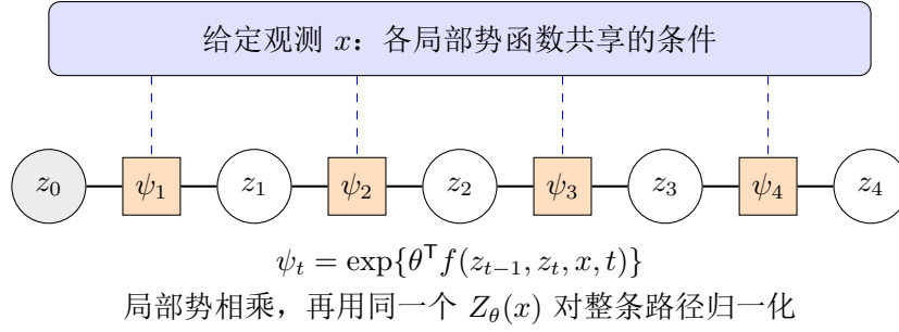
图 7.4: 线性链 CRF 的因子图。圆形表示标签, 方形表示相邻标签的势函数; 实线无方向, 表示变量参与因子。蓝色虚线仅表示势函数依赖已给定观测, 不是标签图中的随机变量边或生成箭头。
