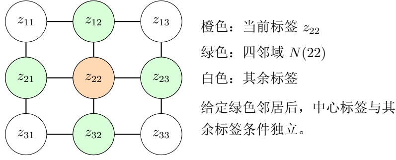
图 7.5: 四邻域网格上的成对 MRF。每个节点对应一个像素或区域标签，每条无向边对应一个二元势；不存在箭头，并不表示各标签独立，而是表示相互作用不采用有向生成分解。
