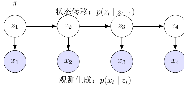
图 7.2: HMM 的有向图结构（以四个时刻为例）。白色圆为隐状态，蓝色圆为已观测变量；横向箭头表示状态转移，向下箭头表示观测生成。箭头表示概率分解关系，不自动代表因果关系。
