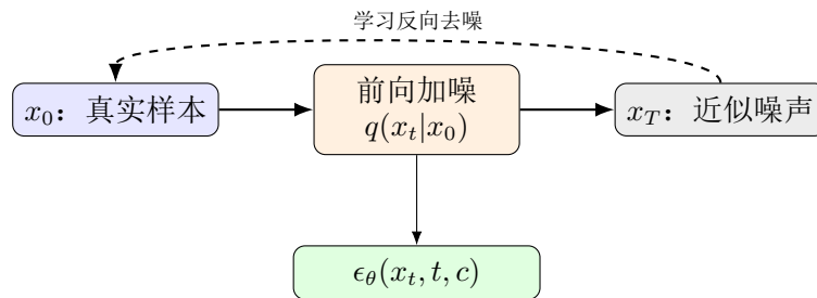
图 13.2: 扩散模型把生成拆为前向加噪和学习反向去噪。
