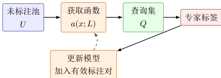
图 18.1: 池式主动学习在每轮用获取函数分配有限标注预算，再用新标签更新模型和下一轮查询。
