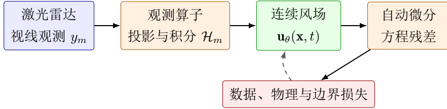
图 14.1: PINN 的信息路径：观测通过测量算子约束场，微分方程和边界条件在未观测位置提供额外约束。
