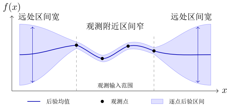
图 8.1: 高斯过程不确定性示意：观测附近的后验区间较窄，远离观测后逐渐变宽。
