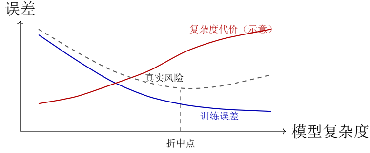
图 6.1: 模型复杂度同时影响拟合误差与估计方差；模型选择的目标是控制真实风险，而不是单独追求训练误差。
