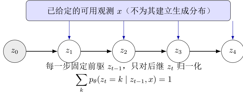
图 7.3: MEMM 的条件有向结构。灰色节点为固定起始状态，观测同时参与各步局部分类；与 HMM 相比，模型不再使用由状态指向观测的生成边。
