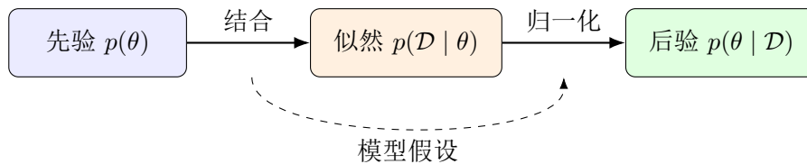
图 7.6: 贝叶斯更新把先验结构与数据证据结合为后验。
