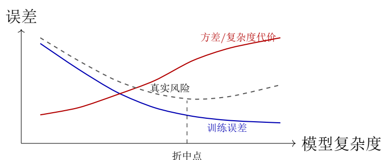
图 7.1: 模型复杂度同时影响拟合误差与估计方差；模型选择的目标是控制真实风险，而不是单独追求训练误差。
