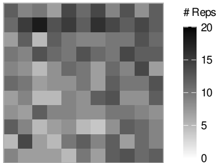
Mistral-7B
