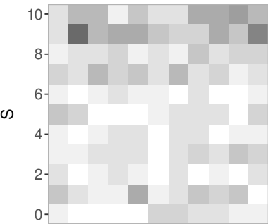
Llama-3.1-8B
