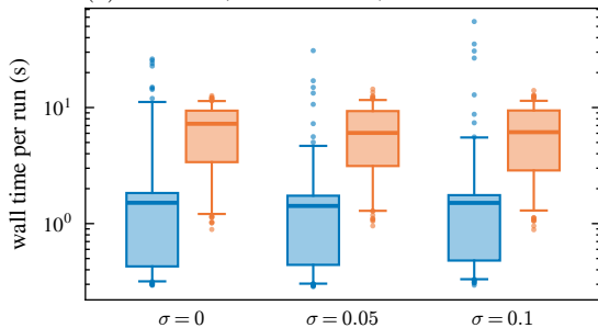
(d) Wall time (one CPU thread)
