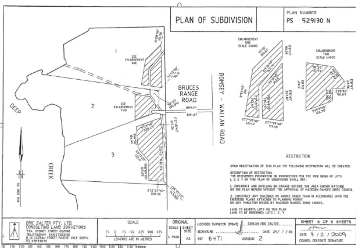
Subdivision Plan – Lots 1,2,3
