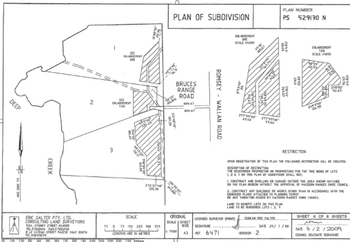
图2: Subdivision Plan – Lots 1, 2, 3
