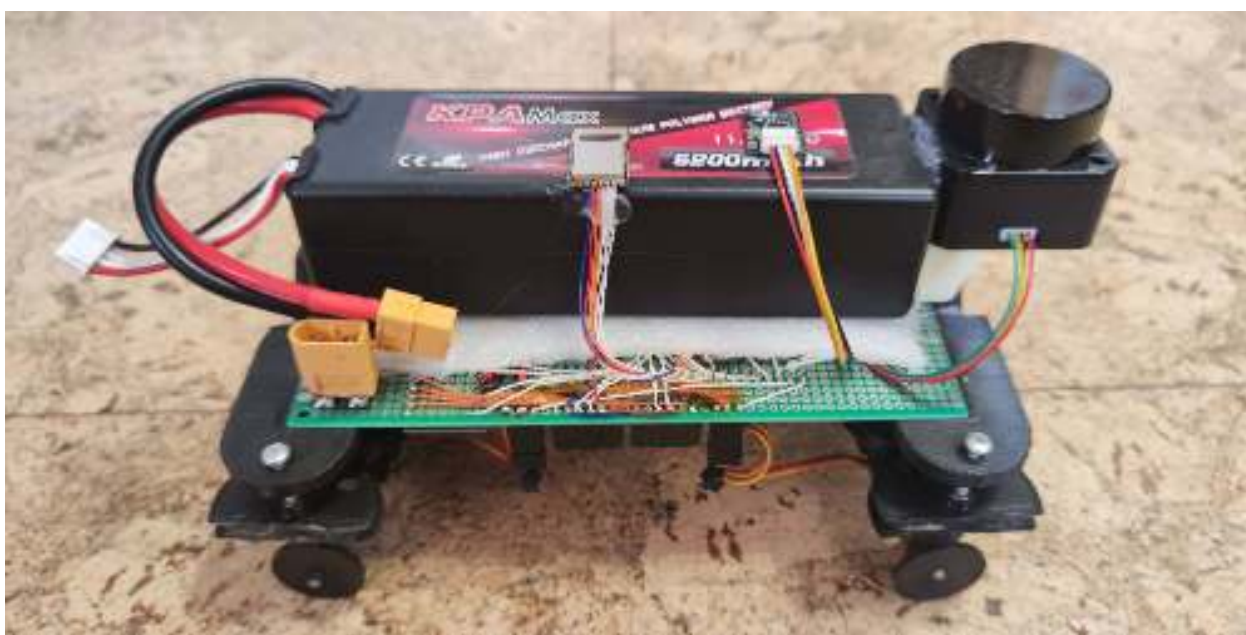
Рисунок 9 – Макет автомобиля
