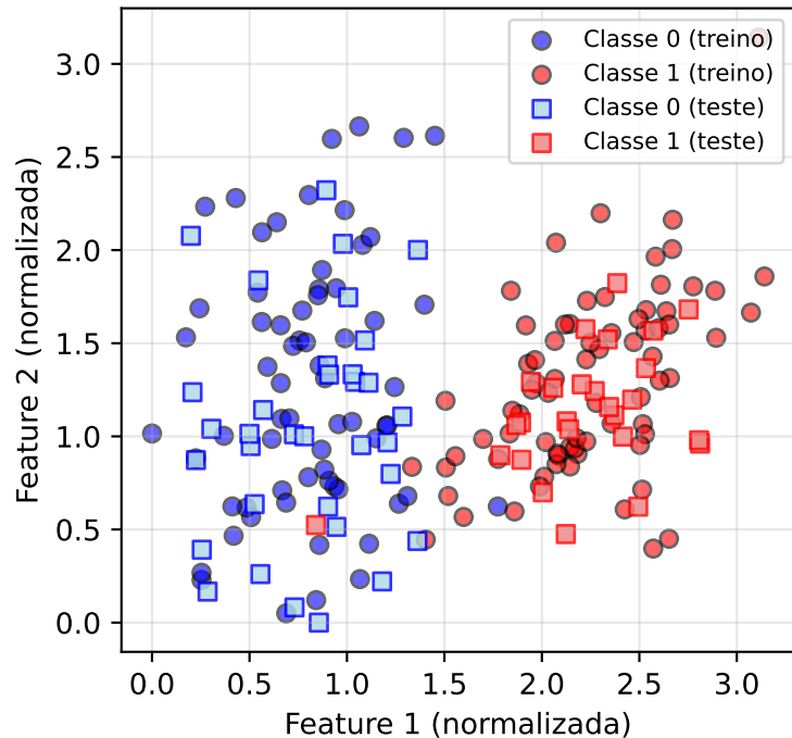
Divisão Treino/Teste
