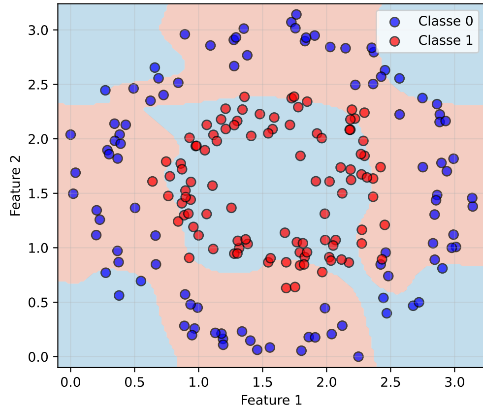
VQC Quântico Acurácia: 0.8500
