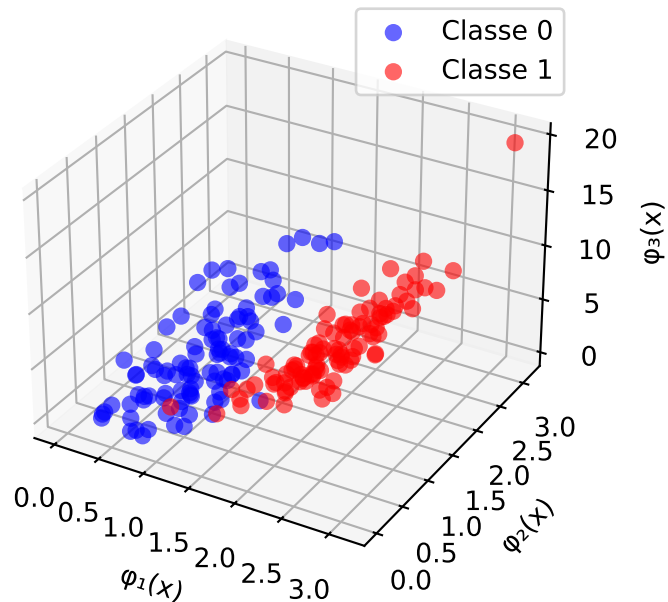
Espaço Transformado (3D)
