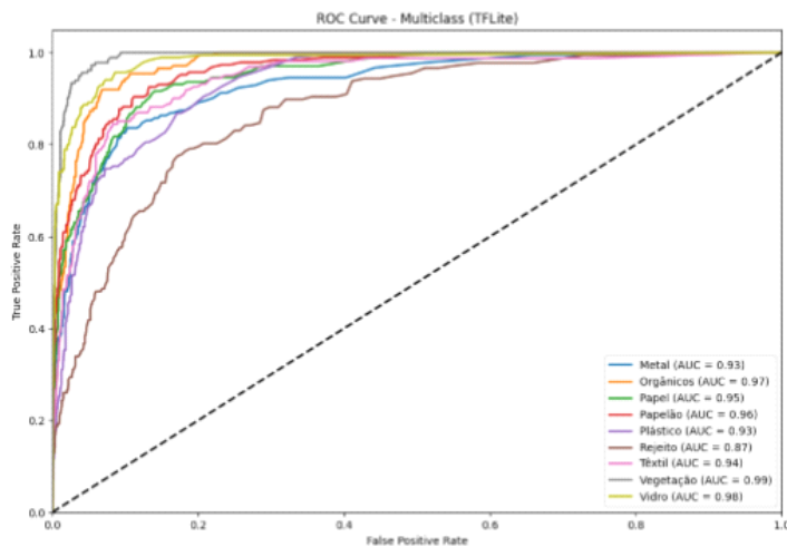
Figura 7: Curvas COR por classe e respectivas AUCs.
