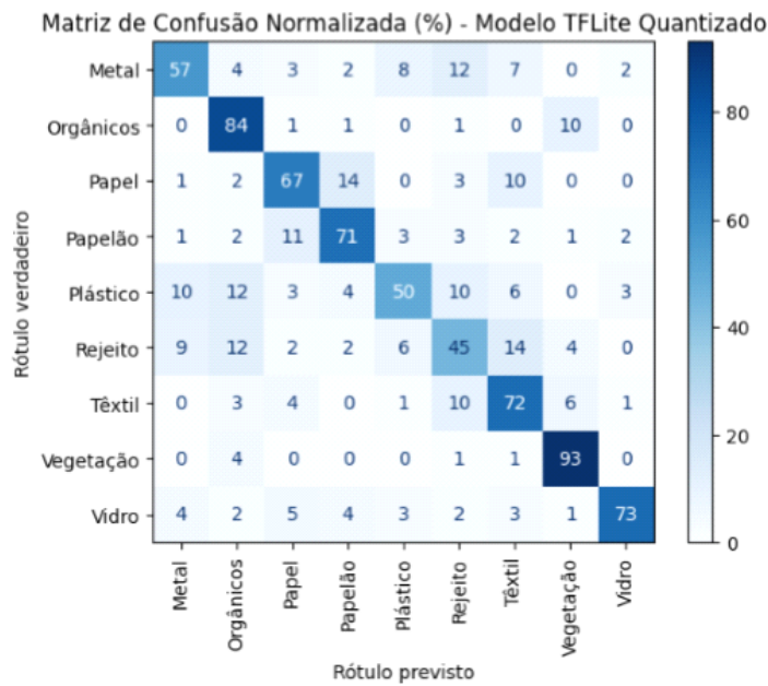
Figura 6: Matriz de confusão normalizada (%).
