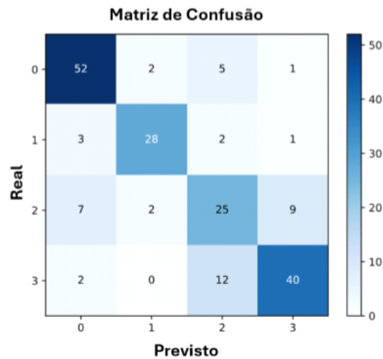
Figura 3: Exemplo de uma Matriz de Confusão.
