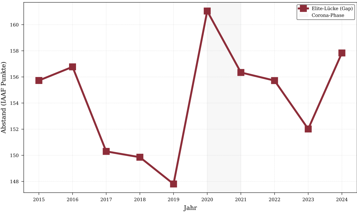
Trend der Elite-Lücke (Abstand Platz 1 zu Verfolgergruppe)
