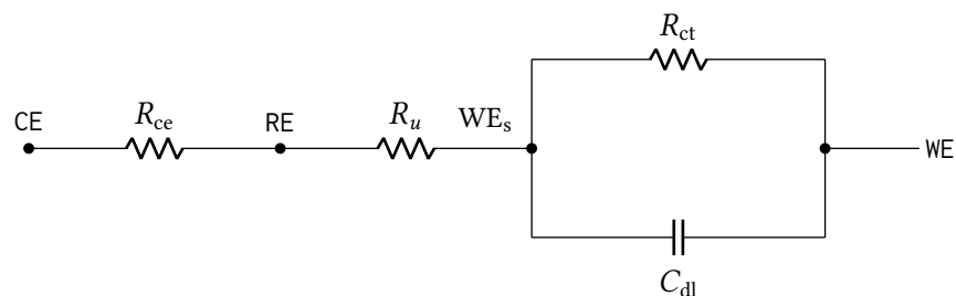
(a) randles_cell
