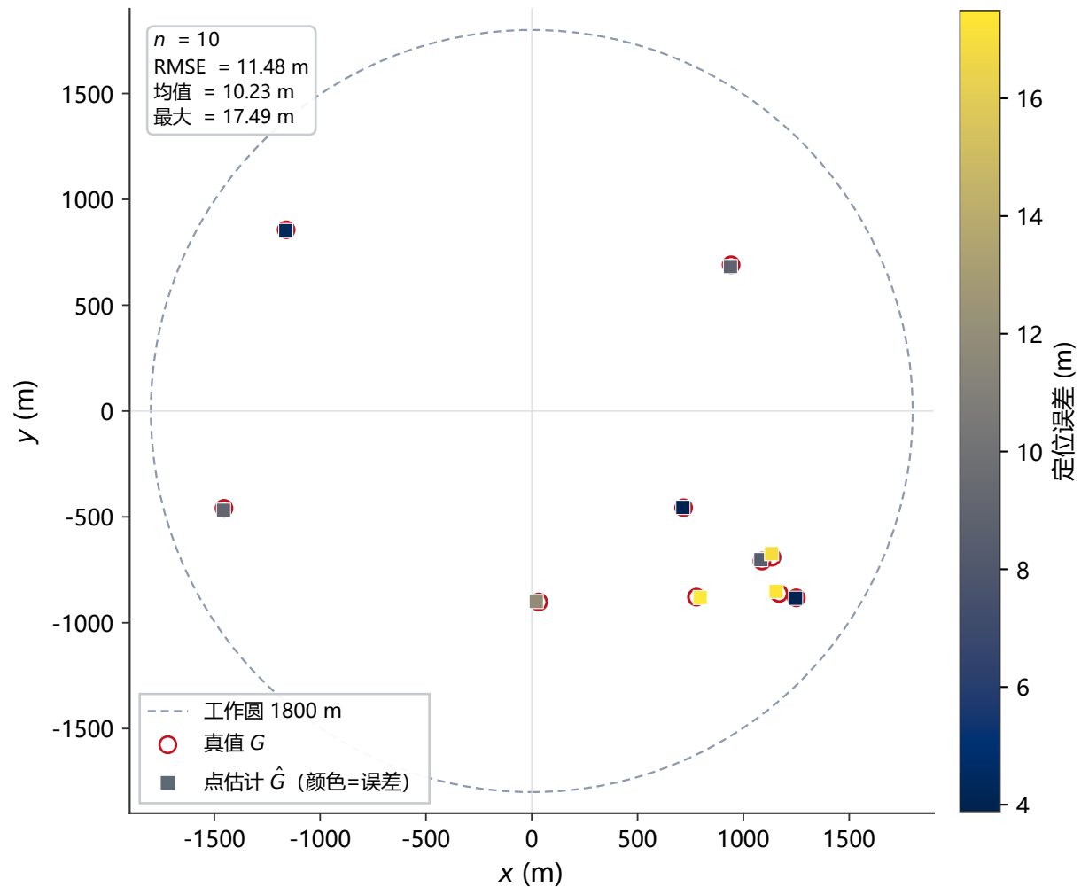
点估计与真值对照
